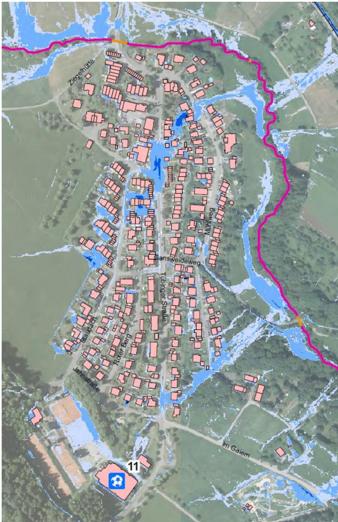
Auswirkungen von außergewöhnlichem Starkregen in Weil im Schönbuch zur Veranschaulichung. Dies ist das Ergebnis einer Vorab-Simulation vom Ingenieurbüro mit möglichen Hochwasserbereichen in Blau.
